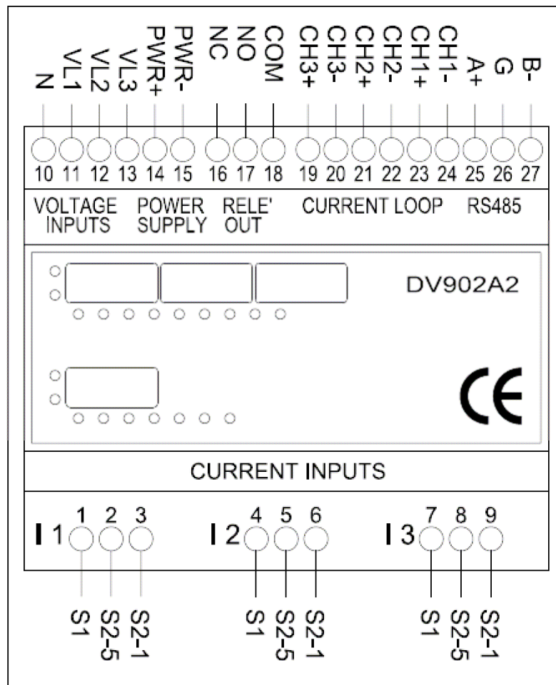
Figura 1 numerazione e nomenclatura morsetti DV902A2
