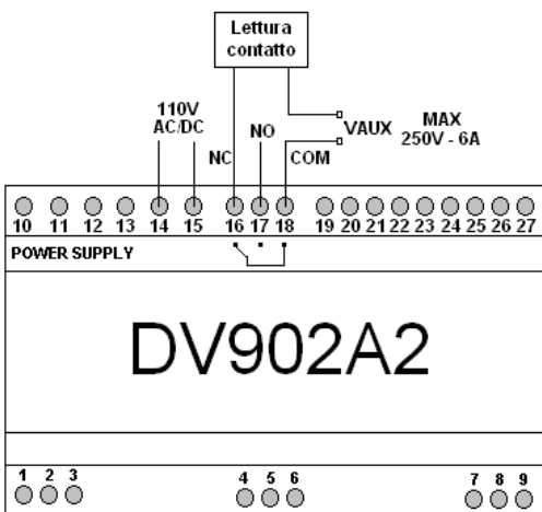
Connessione uscita digitale a relè (esempio per collegamento su NC)
