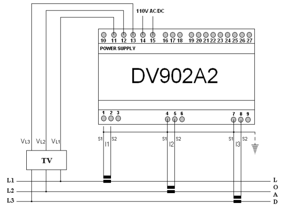
Connessione trifase senza neutro con 3TA e 3TV
