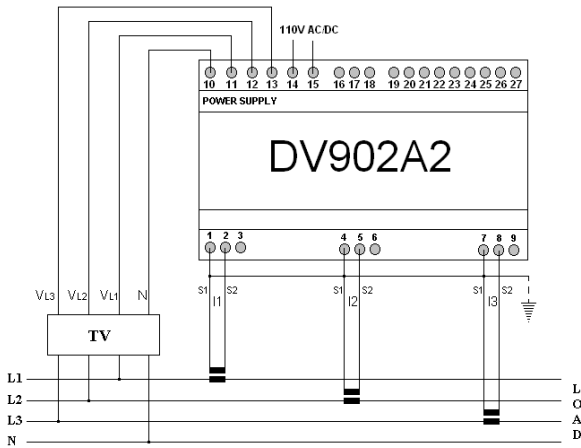
Connessione trifase con 3 TA e 3TV
