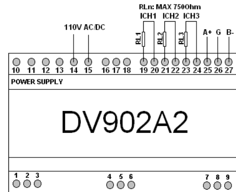
Connessione uscite analogiche e Interfaccia RS485
