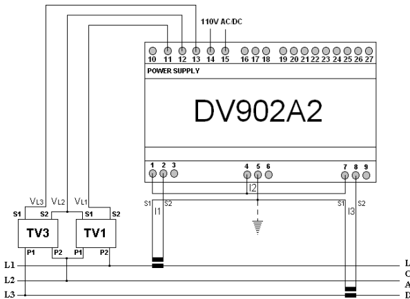
Connessione trifase senza neutro con 2TA e 2TV
